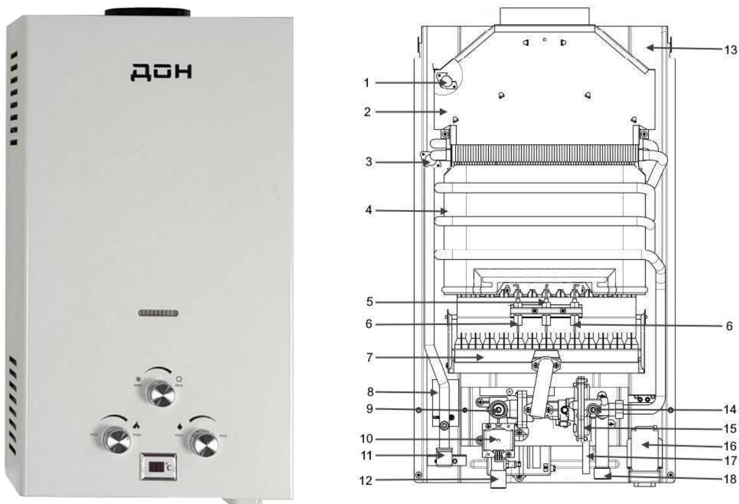
Рис. 1. Аппарат водонагревательный проточный газовый бытовой
