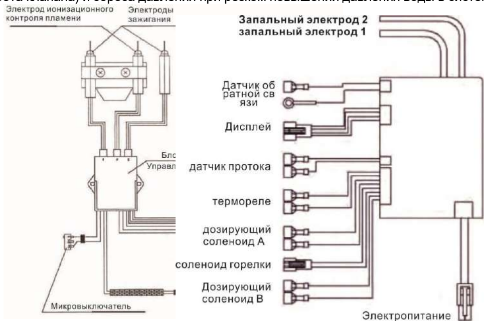
Рис. 2. Схема электрическая
