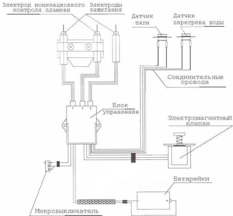
Рис. 2. Схема электрическая
